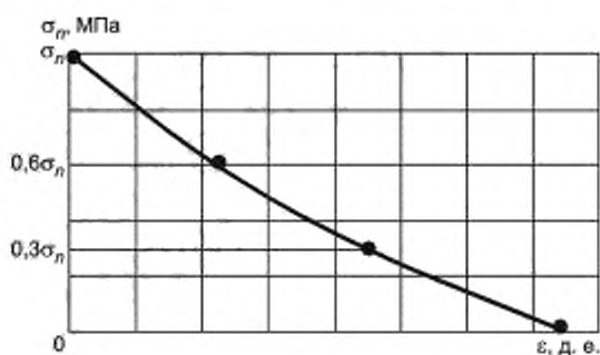
Рисунок В.1 — График зависимости относительной деформации пучения \varepsilon от нормальной силы морозного пучения \sigma
