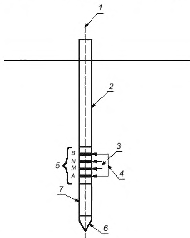
1 — ось зонда; 2 — штанга зонда; 3 — приемные электроды; 4 — питающие электроды; 5 — блок электродов; 6 — конус; 7 — муфта крепления
