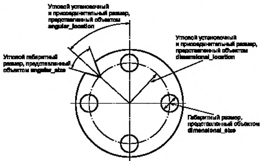
Рисунок 12 — Установочный и присоединительный размер и габаритный размер
