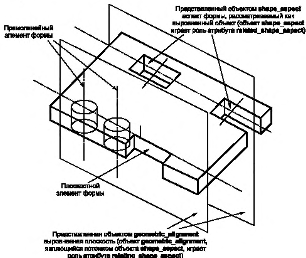
Рисунок 5 — Выравнивание геометрических элементов
