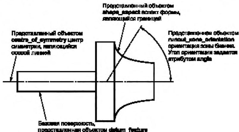
Рисунок 14 — Определение поля допуска биения
