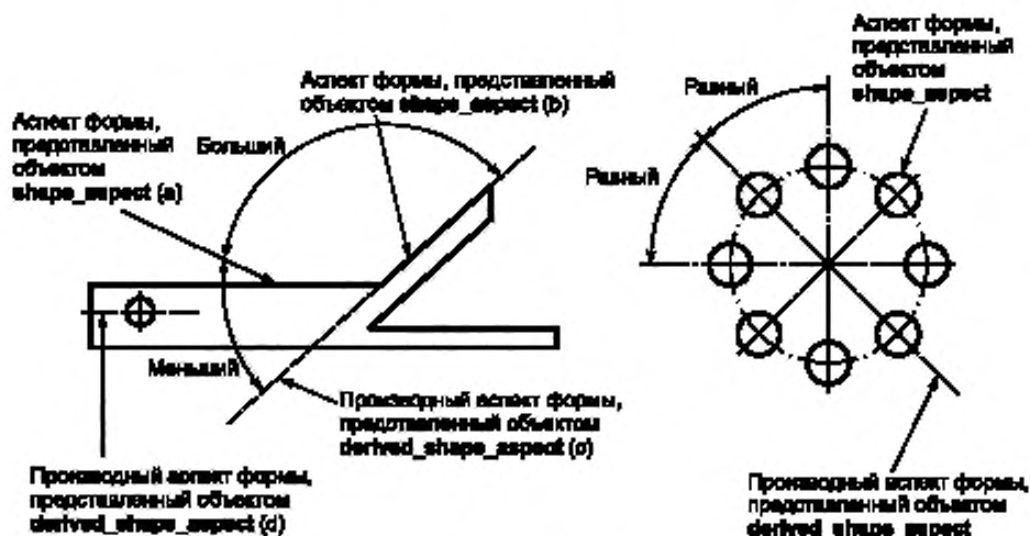
Рисунок 10 — Угловые установочные и присоединительные размеры
