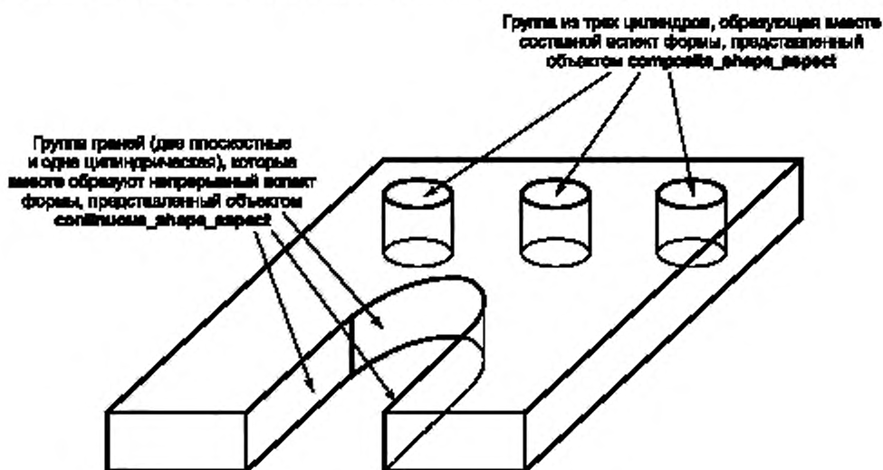
Рисунок 3 — Составной аспект формы
