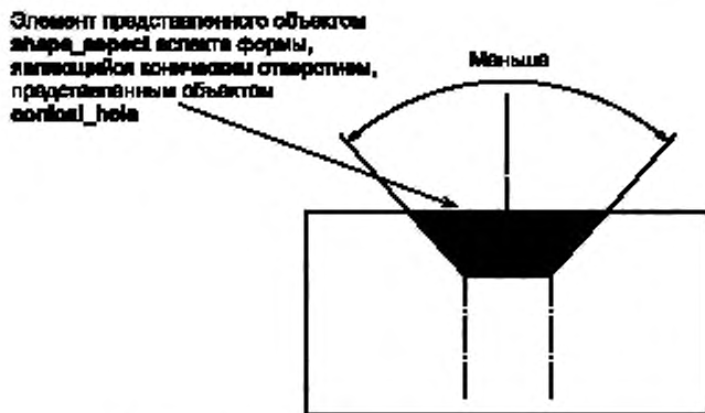
Рисунок 9 — Единичный угловой аспект формы
