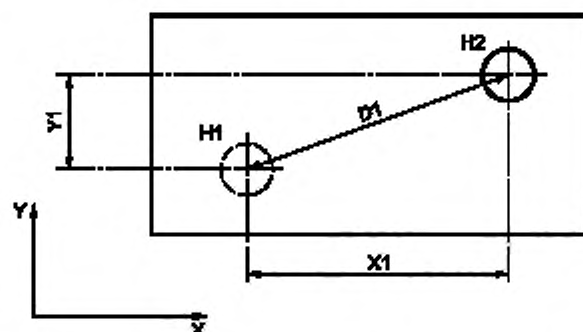
Рисунок 13 — Установочный и присоединительный размер с измеряемым отрезком
