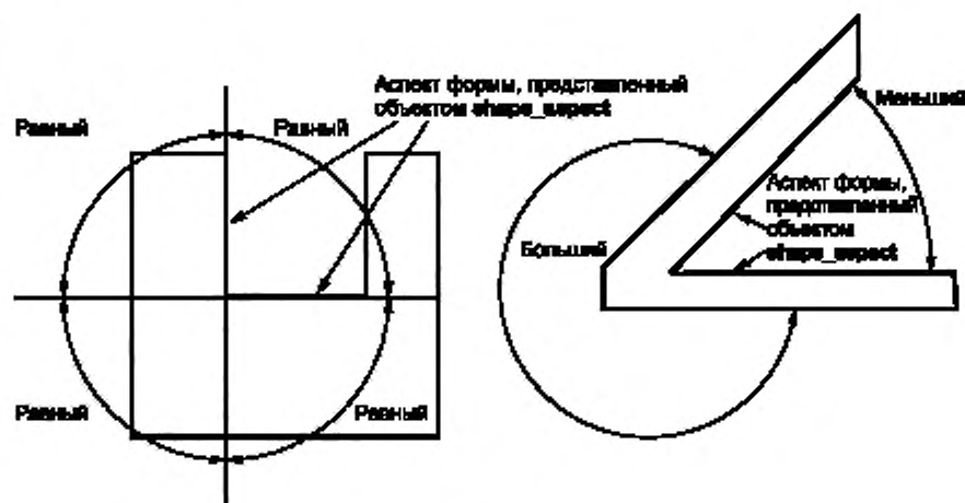
Рисунок 11 — Угловой габаритный размер
