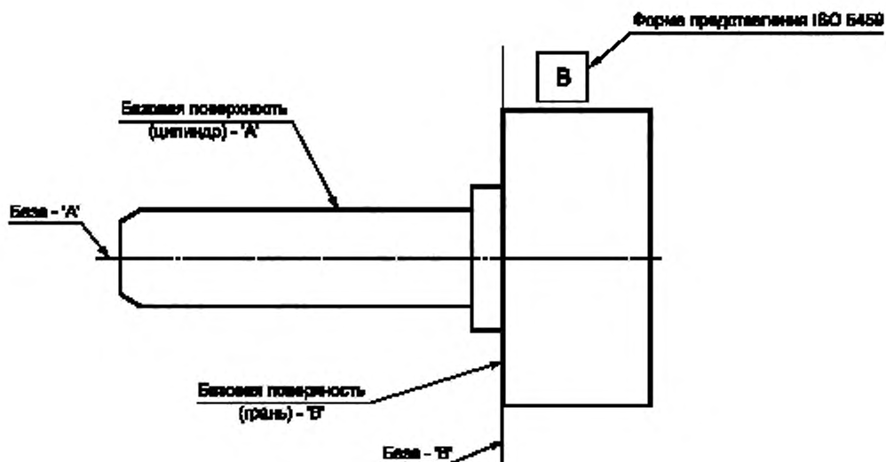
Рисунок 4 — Пример базы и базовой поверхности
