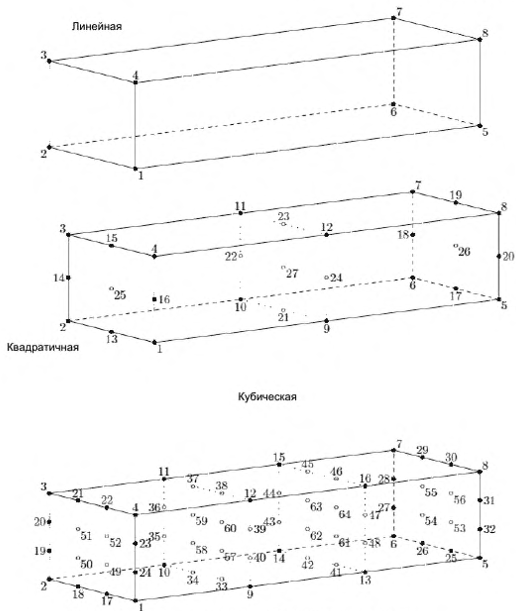
Рисунок 17 — Линейные, квадратичные и кубические шестигранные ячейки
