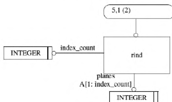
Рисунок D.5 — Представление схемы mesh_topology_schema на уровне объектов в формате EXPRESS-G (5 из 10)
