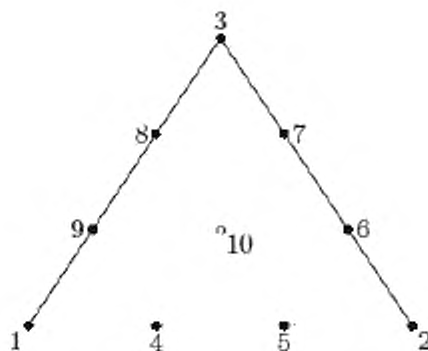
Рисунок 15 — Линейные, квадратичные и кубические треугольные ячейки
