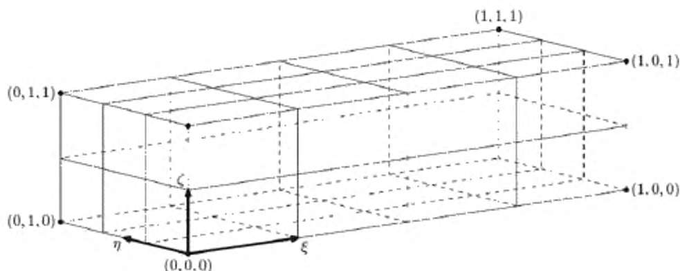
Рисунок 13 — Параметрическая система координат для трехмерной структурированной сетки
