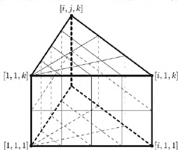
Рисунок 8 — трехмерная пятигранная сетка (при значениях i = 5 , j = 4 , k = 3 )
