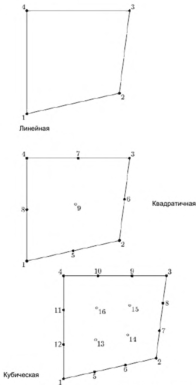
Рисунок 16 — Линейные, квадратичные и кубические четырехугольные ячейки
