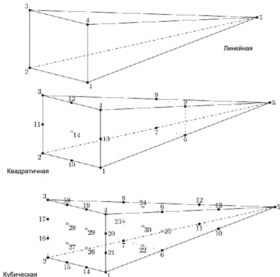
Рисунок 20 — Линейные, квадратичные и кубические пирамидальные ячейки
