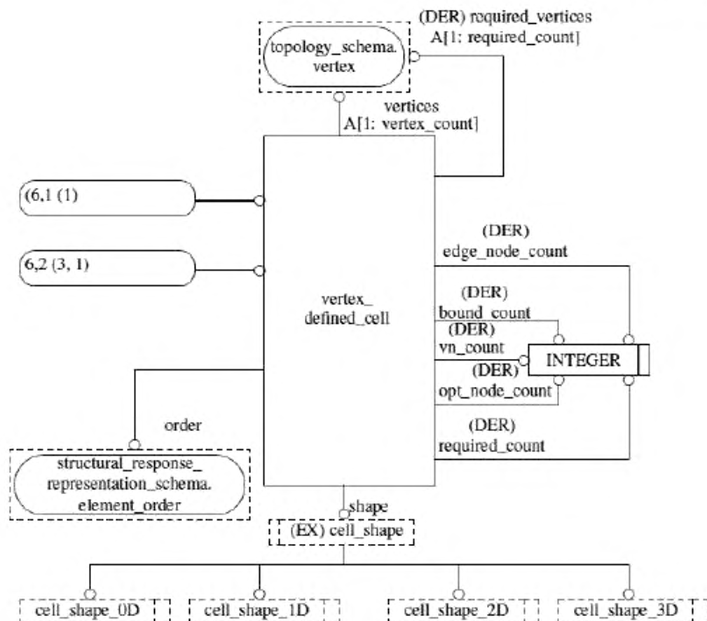
Рисунок D.6 — Представление схемы mesh_topology_schema на уровне объектов в формате EXPRESS-G (6 из 10)
