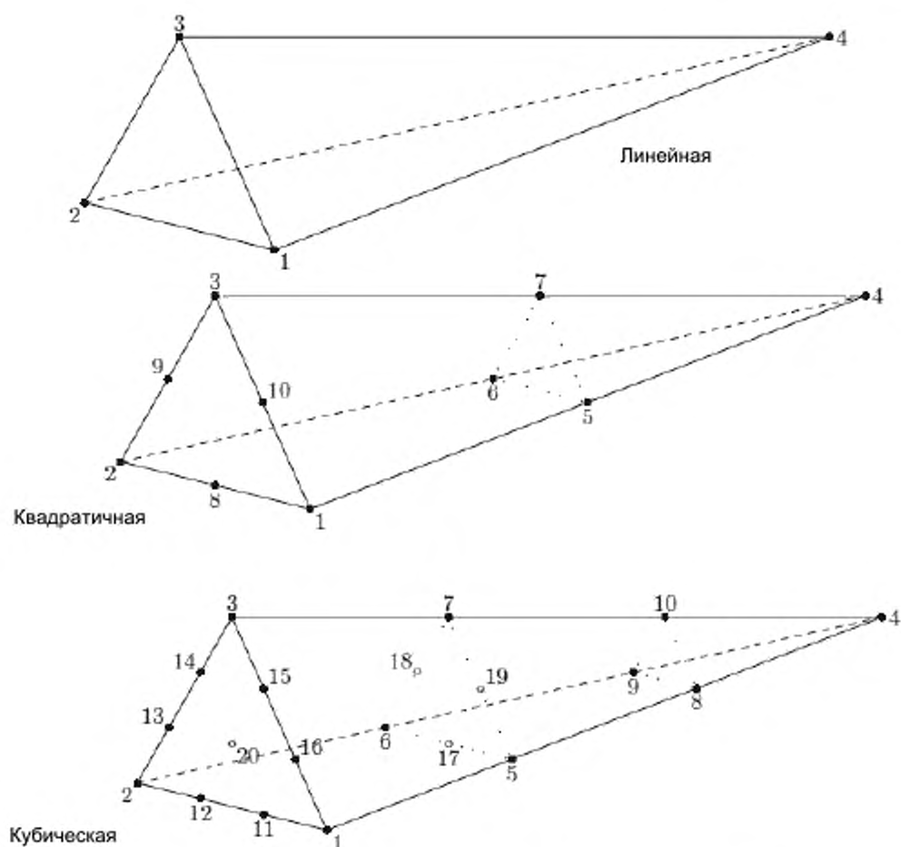
Рисунок 19 — Линейные, квадратичные и кубические тетраэдральные ячейки
