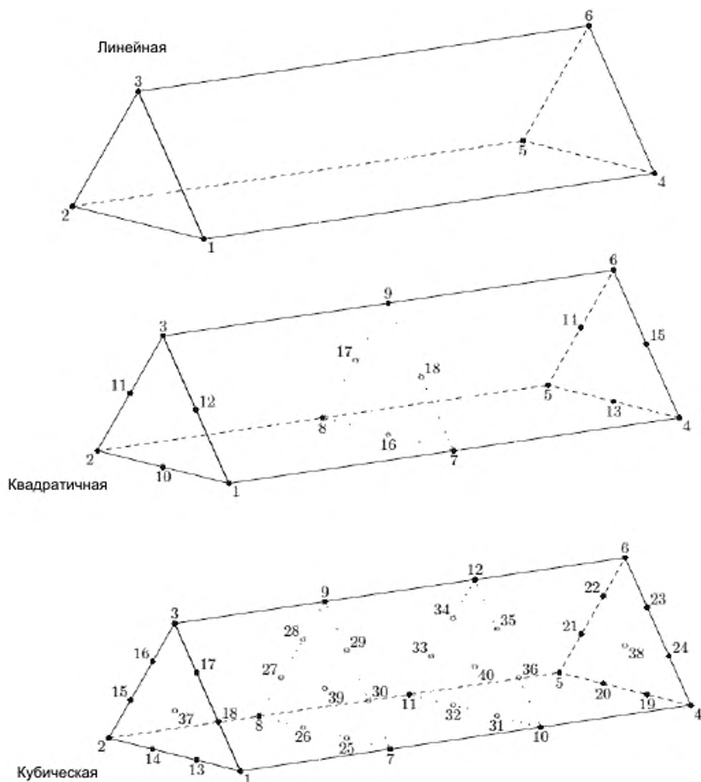
Рисунок 18 — Линейные, квадратичные и кубические клиновидные ячейки
