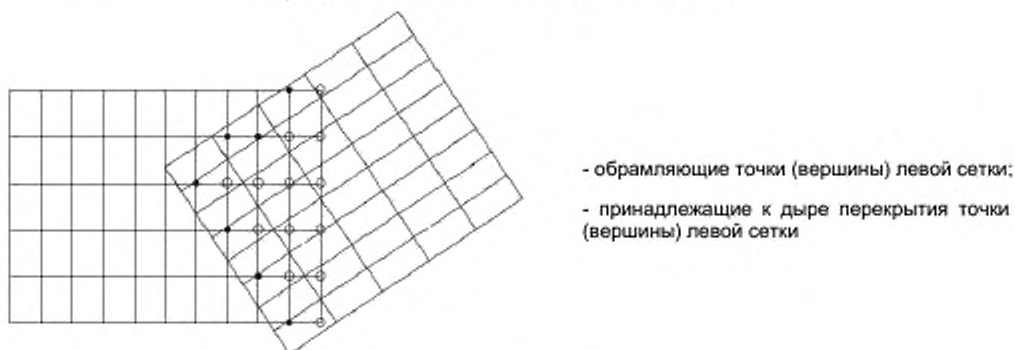
Рисунок 23 — Стык с перекрытием
