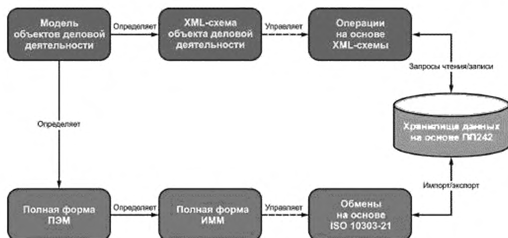
Рисунок Н.2 — Модели и реализации протокола ПП242
