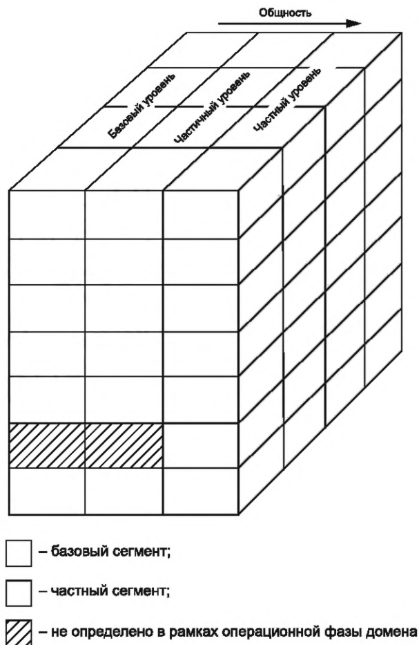
Рисунок 3 — Размерность общности
