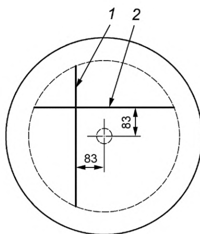
Рисунок 2 — Пример монтажа зоны испытания на пригодность для роликовых ступьев (рулоны, плитки и пластины)
