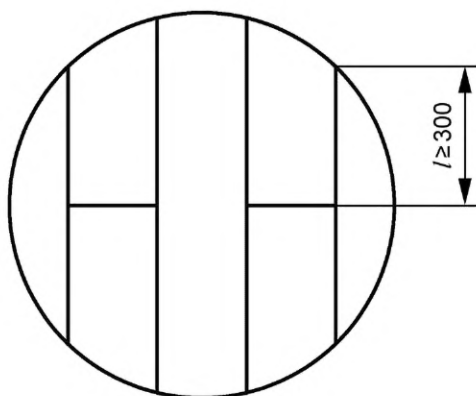
Рисунок 1 — Пример монтажа зоны испытания на пригодность для роликовых ступьев (пластины)
