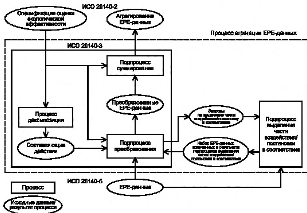
Рисунок 2 — Процесс агрегации EPE-данных
