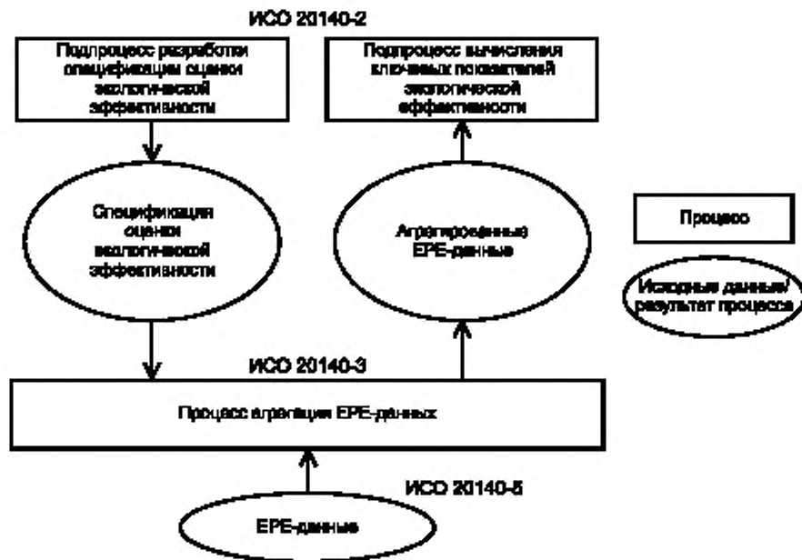
Рисунок 1 — Роль процесса агрегации ЕРЕ-данных
