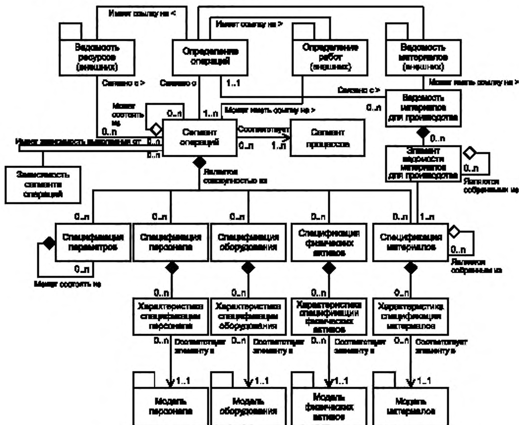
Рисунок A.7 — Модель определения операций (МЭК 62264-2)
