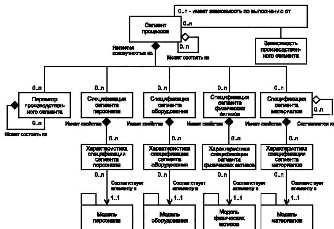
Рисунок А.6 — Модель производственного сегмента (МЭК 62264-2)
