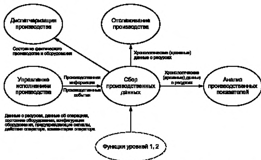
Рисунок А.4 — Интерфейсы функциональной модели сбора производственных данных (МЭК 62264-3)
