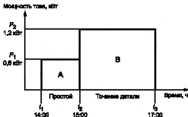
Рисунок В.1 — Статистика энергопотребления металлорежущего станка
