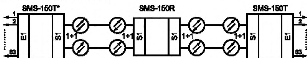
Б.1 Система передачи 155 Мбит/с
