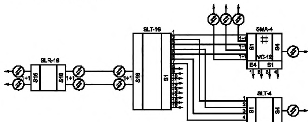
Рисунок Б.3 — Система передачи 2,5 Гбит/с
