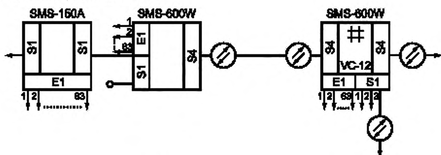
Рисунок Б.2 — Система передачи 622 Мбит/с
