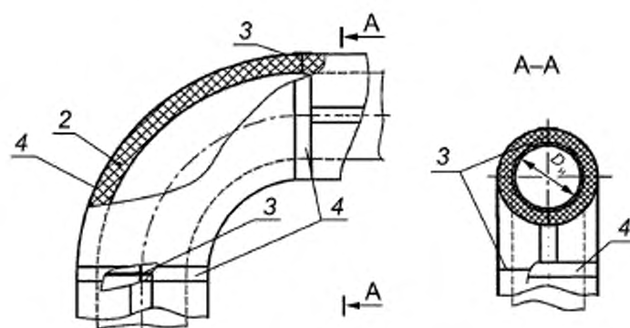
б) Изоляция отвода термоизоляционными листами ( D_{\text{н}} > 160 мм)
