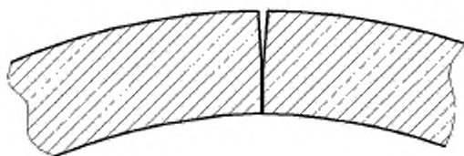
б) Частичный непровар при высокочастотной сварке
