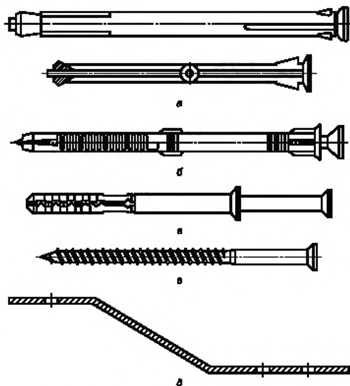
Рисунок Б.1 — Примеры крепежных элементов
