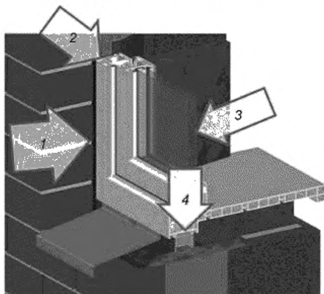
1 — внешние воздействующие факторы; 2 — механические силы, действующие на конструкции; 3 — параметры микроклимата помещений; 4 — эксплуатационные нагрузки
