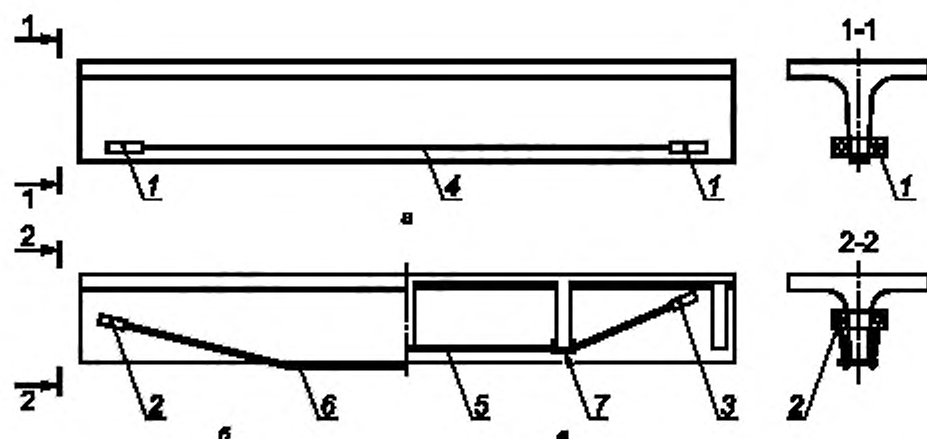
1—3 — анкерные узлы различной конструкции; 4 — прямолинейные и 5 — полигональные шпренгели (напрягаемые затяжки), 6, 7 — оттяжки (оггибающие устройства) различной конструкции
