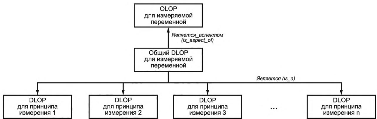
Рисунок 3 — Присвоение OLOP и DLOP оборудованию, используемому для измерения одного типа переменной
