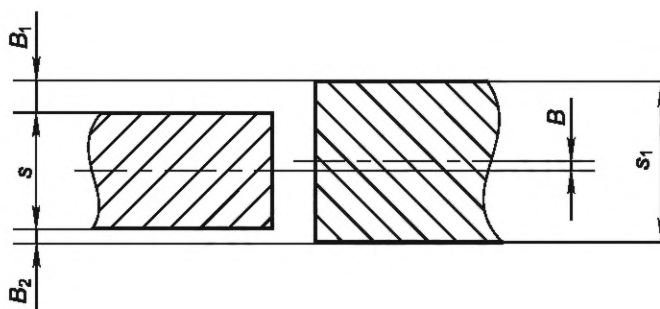
Рисунок 5 — Смещение кромок
