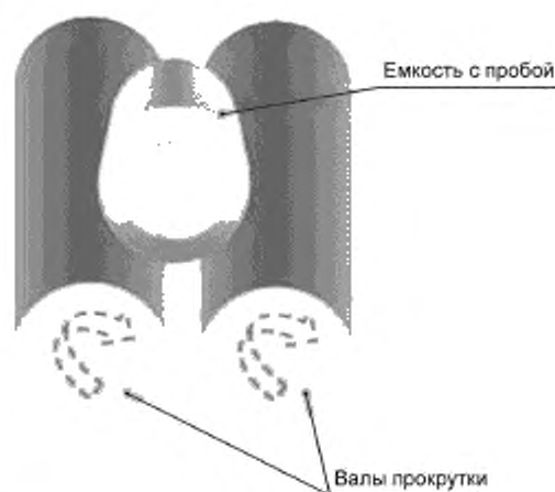
Рисунок А.1 — Схематическое изображение устройства для вращения емкости с пробой
