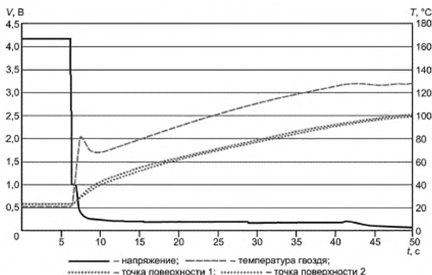
Рисунок 5 — График зависимости напряжения и температуры от времени для одиночного испытываемого образца
