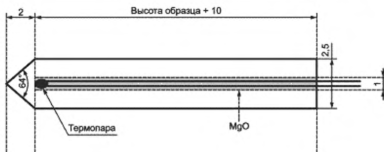
Рисунок 1 — Схематическое изображение испытательного гвоздя
