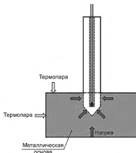
Рисунок 2 — Схематическое изображение испытательного гвоздя и нагретого металлического бруска
