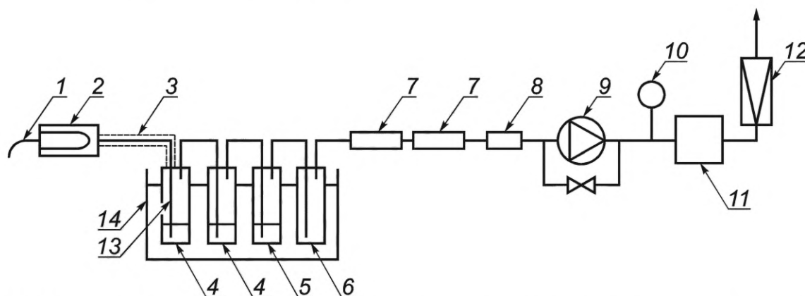
1 — пробоотборный зонд; 2 — собранный фильтр; 3 — линия передачи с подогревом; 4 — импинджер с \text{SnCl}_2 ; 5 — импинджер для очистки газа; 6 — осушающий импинджер (пустой); 7 — золотосодержащая амальгамационная ловушка; 8 — сушильная установка (силикагель); 9 — насос; 10 — термометр и манометр; 11 — газовый счетчик; 12 — расходомер; 13 — сопло импинджера; 14 — охлаждающая ванна
