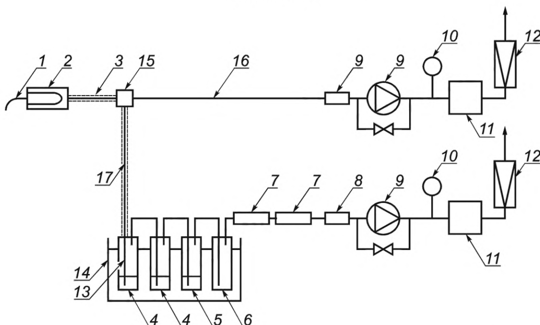
Рисунок 2 — Принципиальная схема основной линии отбора проб с обогреваемой установкой каталитического восстановления
