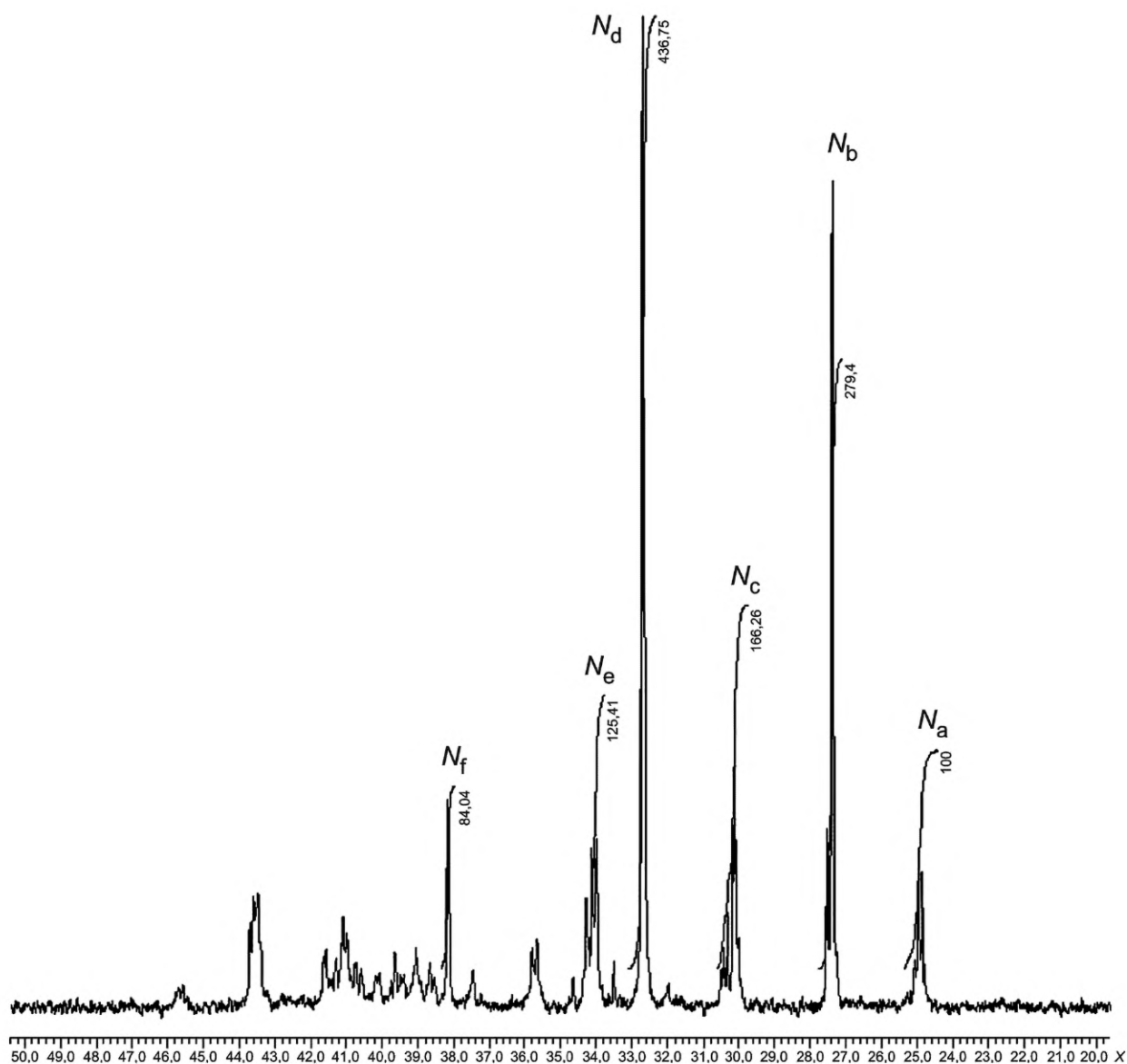
Рисунок С.1 — Пример спектра ^{13}\text{C} ЯМР S-SBR
