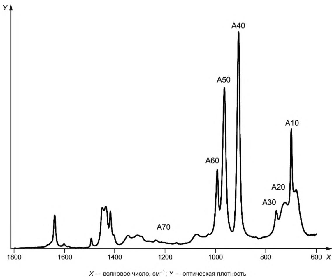
Рисунок 1 — Спектр ATR типичного S-SBR
