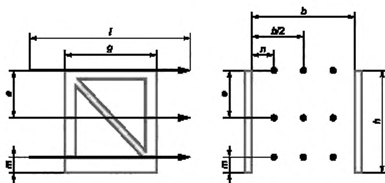
b — ширина ворот; e — расстояние между плоскостями прохода; g — ширина антенны; l — расстояние прохода; h — расстояние до верхней границы области обнаружения; m — расстояние до нижней границы области обнаружения; l — расстояние от плоскости антенны до первых точек измерений
