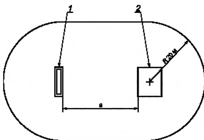
1 — измерительная антенна; 2 — испытуемое устройство (две антенны); a = 10 м, R = 20 м (свободное поле)
