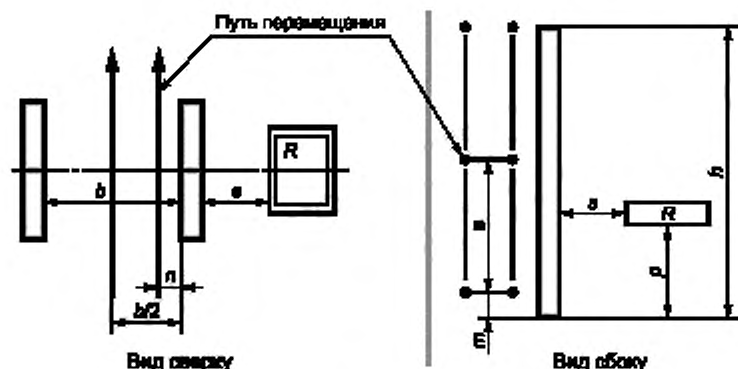
b — ширина ворот; e — расстояние между плоскостями прохода; h — расстояние до верхней границы области обнаружения; m — расстояние до нижней границы области обнаружения; n — расстояние от плоскости антенны до первых точек измерений; p — высота расположения нижней границы рабочей зоны; R — источник помех (петлевая антенна); s — расстояние до источника помех
