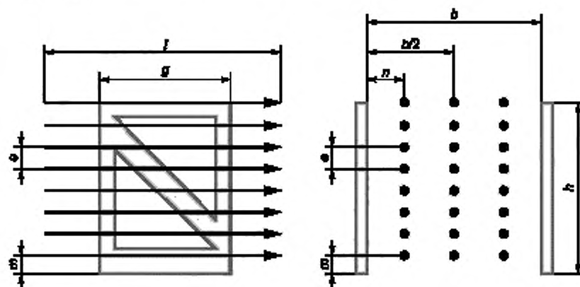
b — ширина ворот; e — расстояние между горизонтальными плоскостями прохода; g — ширина антенны; l — расстояние прохода; h — расстояние до верхней границы области обнаружения; m — расстояние до нижней границы области обнаружения; n — расстояние от плоскости антенны до первых точек измерений.
