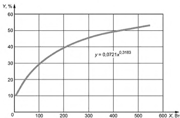
а) Эффективность циркуляционных насосов с гидравлической мощностью, менее или равной 500 Вт (источник: COSTIC)
