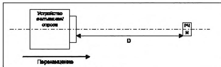
Рисунок 19 — Установка для измерения дальности идентификации, считывания и записи
