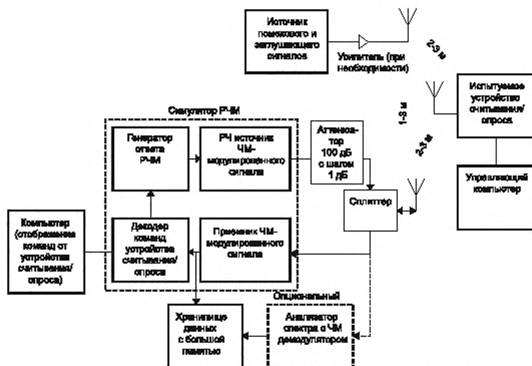
Рисунок 1 — Испытательный стенд для испытаний устройства считывания/опроса по ГОСТ Р ИСО/МЭК 18000-7
