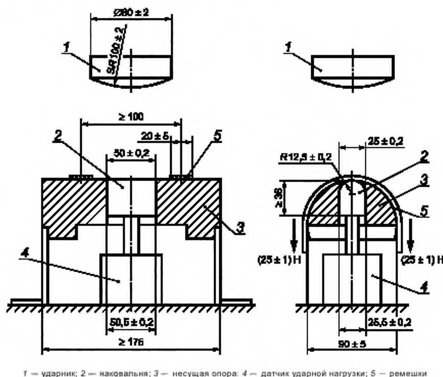
Рисунок 13 — Принцип испытания на удар экипировки для рук и ног
