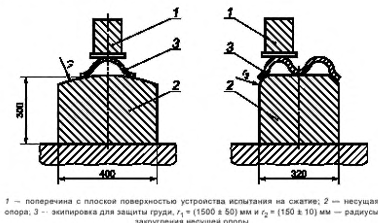
Рисунок 5 — Принцип испытания деформации средства защиты
