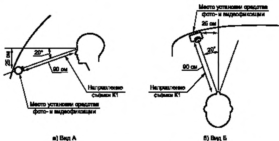
Рисунок А.1 — Принципиальная схема установки СМВ в салоне КТС категорий М, N
