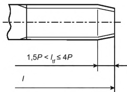
Рисунок 1 — Длина выдавливающего участка
