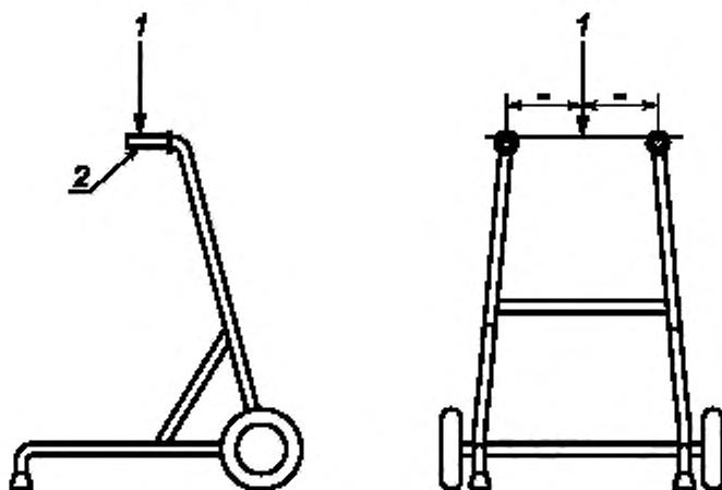
1 — нагрузка, 2 — задняя контрольная точка ручки
