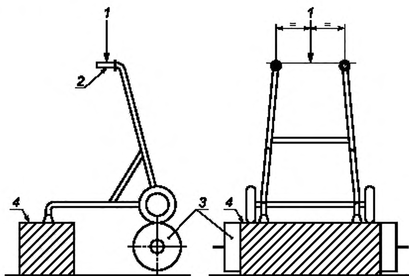
1 — нагрузка, приложенная в контрольной точке, 2 — задняя контрольная точка рукоятки, 3 — движущая поверхность; 4 — неподвижная поверхность
