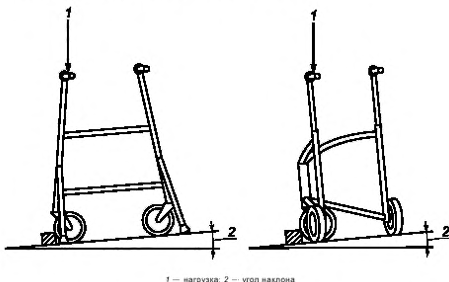
Рисунок 9 — Схема нагружения при испытании на боковую устойчивость
