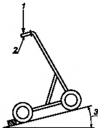
1 — нагрузка; 2 — задняя контрольная точка рукоятки; 3 — угол наклона
