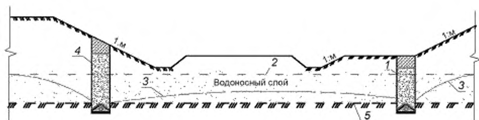
1 — заковетный дренаж, устроенный на полке; 2 — уровень грунтовых вод до понижения; 3 — кривая депрессии после устройства дренажа; 4 — заковетный дренаж, устроенный на откосе выемки; 5 — водоупорный слой
