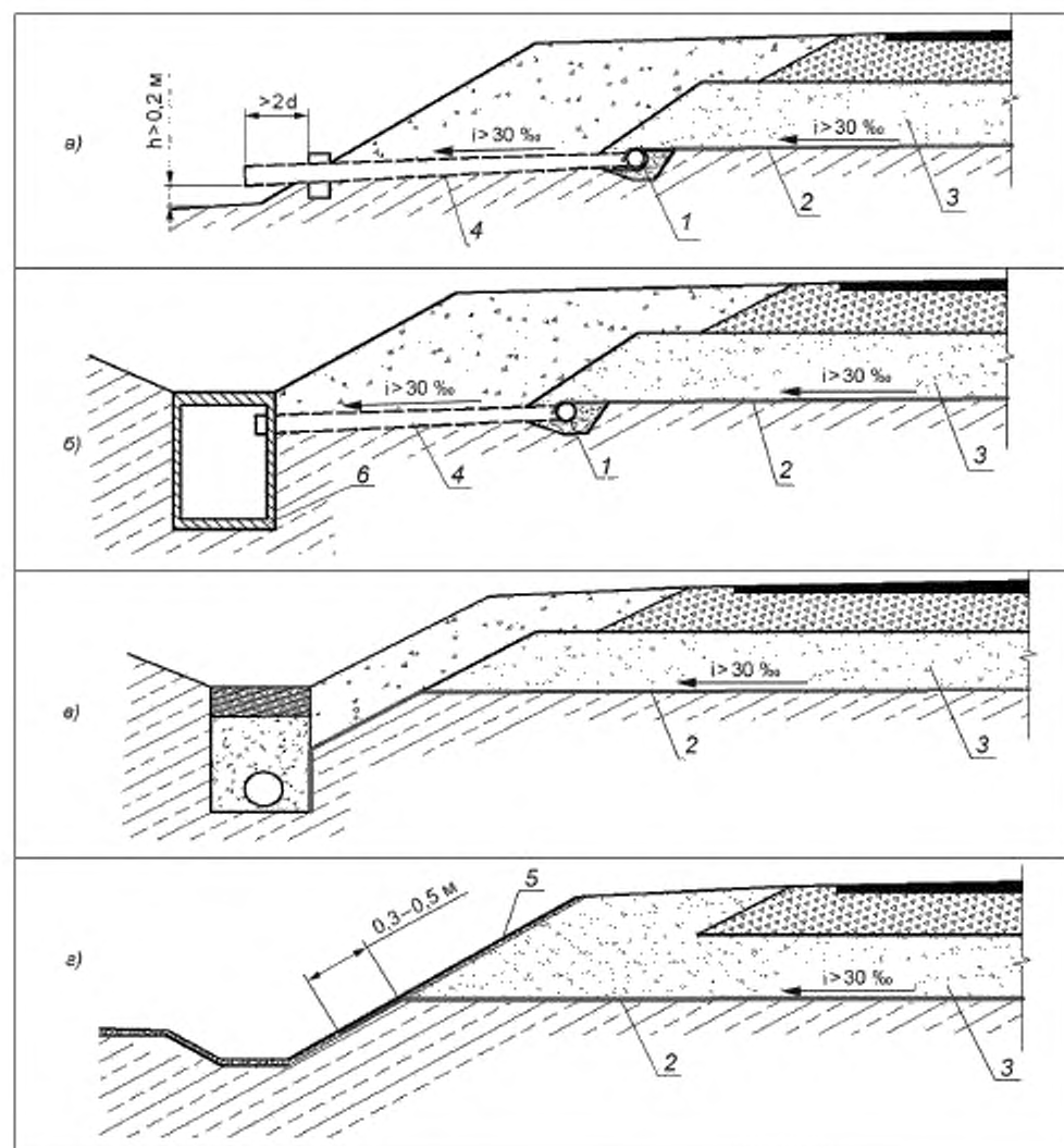
Дренажи с выпуском воды: а) — на рельеф; б) — в закрытый продольный поток; в) — в трубчатый дренаж; г) — на откос насыпи 1 — продольная дренажная труба, 2 — геокomпозитный дренаж, 3 — песчаный дреннрующий и технологический защитный слой с K_{\text{ф}} \geq 0,5 м/сут; 4 — дренажные трубы поперечных выпусков; 5 — растительный слой на откосе насыпи; 6 — закрытый продольный поток
