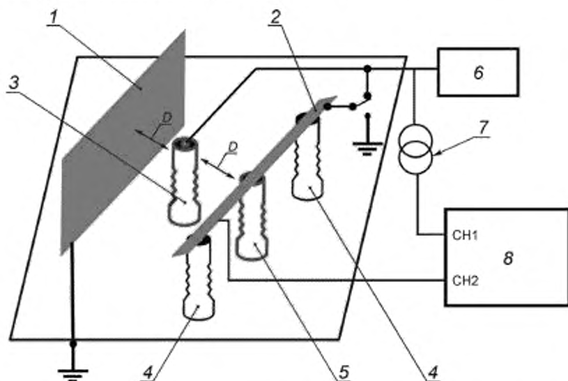
1 -- металлическая стенка; 2 -- шина; 3 -- объект испытания, испытываемое оборудование; 4 -- изолирующая опора; 5 -- ММТН; 6 -- высоковольтный генератор; 7 -- эталонный ТН; 8 -- измерительный прибор. D -- расстояние между фазами
