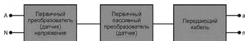
Рисунок 1101 — Общая блок-схема однофазного пассивного ММТН
