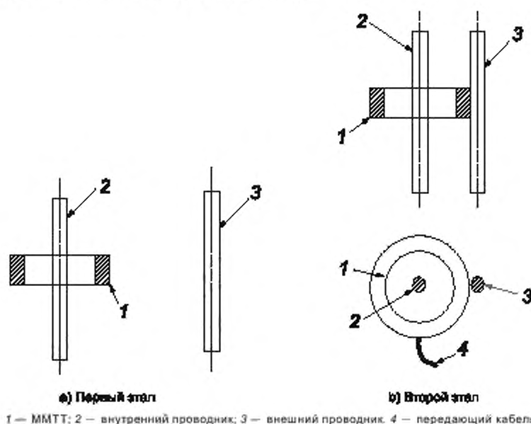
Рисунок 1003 — Испытательная установка для проверки влияния магнитного поля на другие фазы
