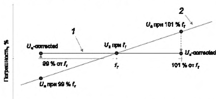
Рисунок 10B.3 — Испытание катушки Роговского на частотную зависимость
