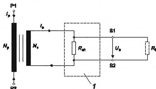
1 — преобразователь ток — напряжение ( R_{sh} является составным компонентом ММТТ). I_p — первичный ток; R_{sh} — шунтирующее сопротивление; U_s — вторичное напряжение; N_p — количество витков первичной обмотки; N_s — количество витков вторичной обмотки; R_b — нагрузка, Ом; P1, P2 — первичные входы; S1, S2 — вторичные выходы
