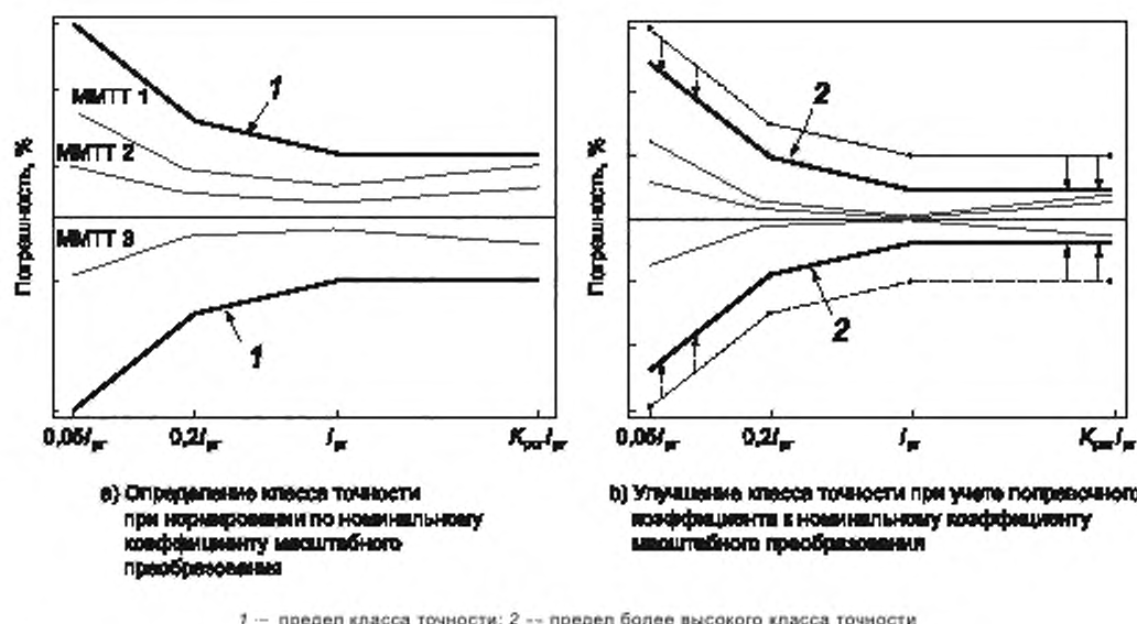
Рисунок 10А.1 — Улучшение класса точности в сторону повышения при использовании поправочного коэффициента CF_I
