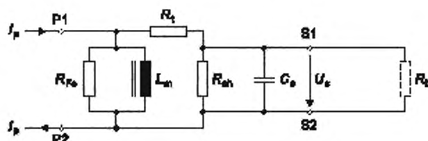
I_p — первичный ток; R_{Fe} — эквивалентное сопротивление потерь; L_m — эквивалентная индуктивность намагничивания; R_t — полное сопротивление вторичной обмотки и проводки; R_{sh} — шунтирующее сопротивление (преобразователь тока в напряжение); C_s — эквивалентная емкость кабеля; U_s — вторичное напряжение; R_b — нагрузка, Ом; P1, P2 — первичные входы. S1, S2 — вторичные выходы
