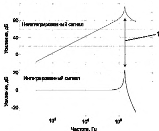
Рисунок 10B.2 — Интегрированные и неинтегрированные выходные сигналы катушки Роговского
