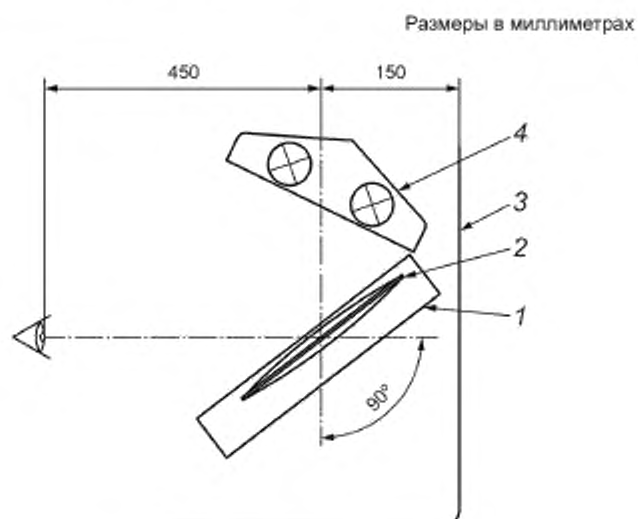
1 — контрольный образец яркости; 2 — испытуемый образец; 3 — матово-черный экран; 4 — лампа
