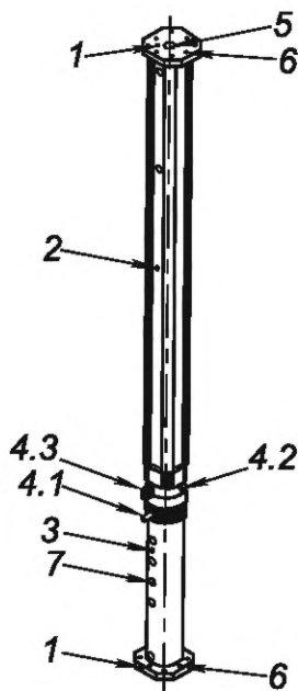
1 — торцевая пластина; 2 — внешняя трубка; 3 — внутренняя трубка; 4.1 — прикрепленный штифт; 4.2 — накидная гайка; 4.3 — рукоять; 5 — центральное отверстие; 6 — соединительные отверстия; 7 — отверстие для штифта
