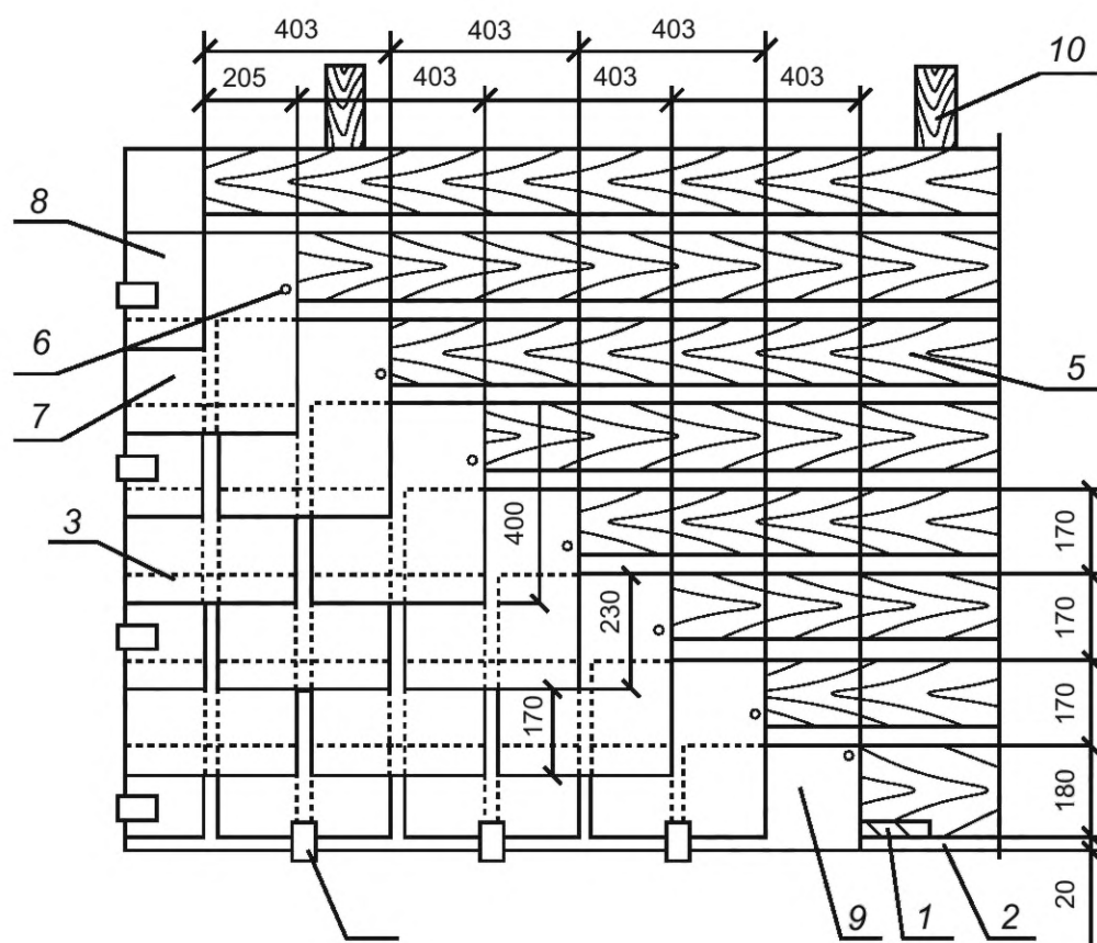
1 — уравнивательная рейка; 2 — свес карниза 20 мм; 3 — разбивочные линии; 4 — противоветровая скоба; 5 — дощатый настил; 6 — гвоздь (саморез); 7 — рядовая плитка; 8 — фризровая плитка; 9 — краевая плитка; 10 — стропило
