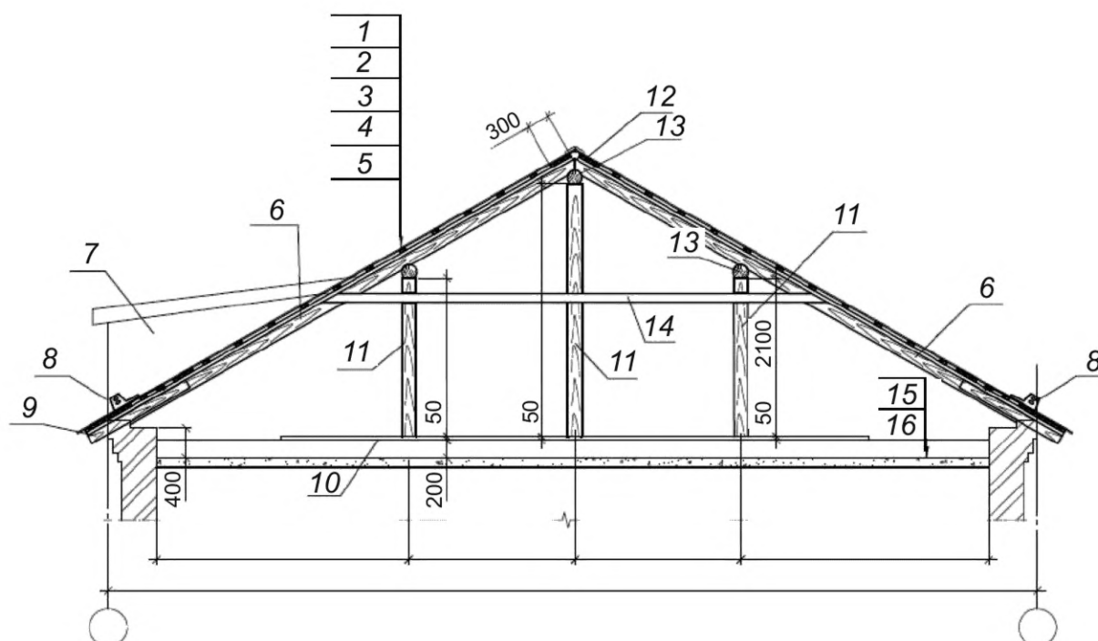
1 — хризотилцементные листы; 2 — обрешетка; 3 — контробрешетка; 4 — водозащитная пленка; 5 — стропильная система; 6 — стропильная нога; 7 — слуховое окно; 8 — элемент системы снегозадержания; 9 — кобылка; 10 — лежень (доска); 11 — стойка; 12 — сплошная обрешетка; 13 — прогон; 14 — затяжка; 15 — теплоизоляция; 16 — перекрытия
