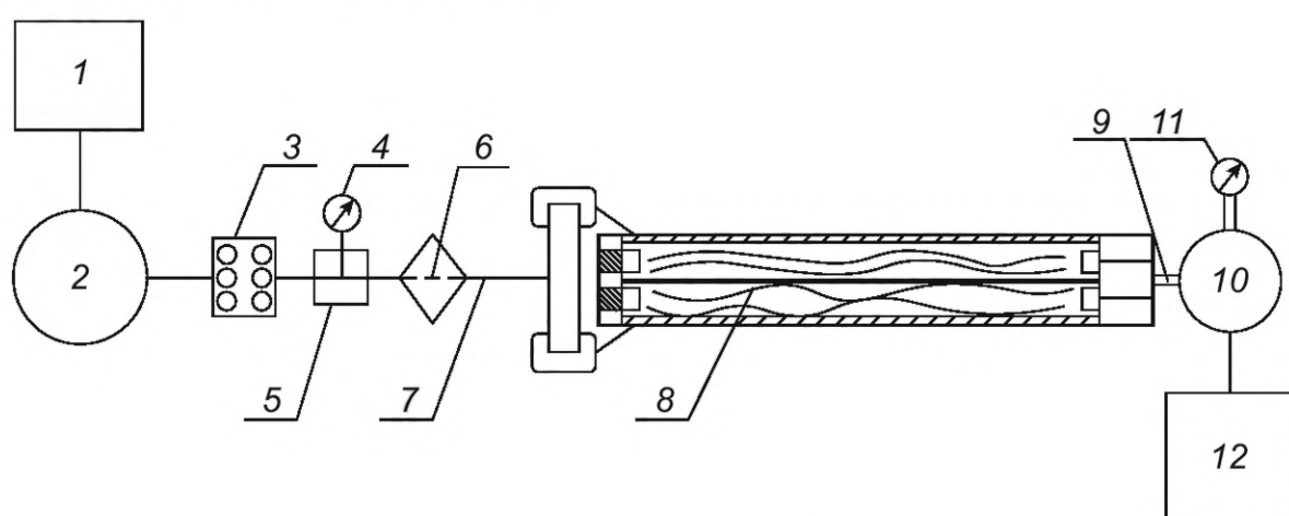
1 — емкость с антисептиком; 2 — насос; 3 — коллектор; 4 — манометр; 5 — гидрораспределитель для разделения потока пропиточного раствора; 6 — фильтр; 7 — трубопровод; 8 — пропиточная установка УПМ; 9 — вакуумный шланг; 10 — вакуум-насос для ускорения процесса пропитки древесины; 11 — вакуумметр; 12 — емкость для сбора жидкости
