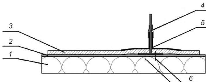
Рисунок 1 — Схематичное изображение устройства слоя
