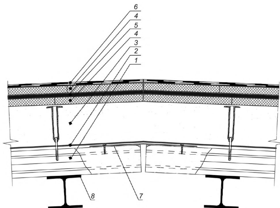
1 — несущая конструкция; 2 — пароизоляция; 3 — теплоизоляция; 4 — листы сборной стяжки; 5 — слой; 6 — покрытие; 7 — уголок из оцинкованной стали; 8 — основание для устройства кровли
