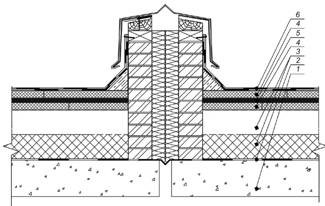
1 — основание для устройства кровли; 2 — пароизоляция; 3 — теплоизоляция; 4 — листы сборной стяжки; 5 — слой; 6 — покрытие
