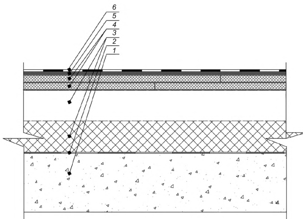
1 — основание (цементная стяжка, бетонная плита и т. п.); 2 — пароизоляция; 3 — теплоизоляция; 4 — уклонообразующий материал; 5 — слой; 6 — покрытие
