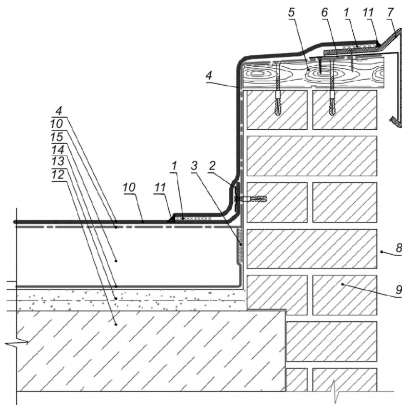
Рисунок Б.7 — Схема монтажа слоя вблизи слива через парапет
