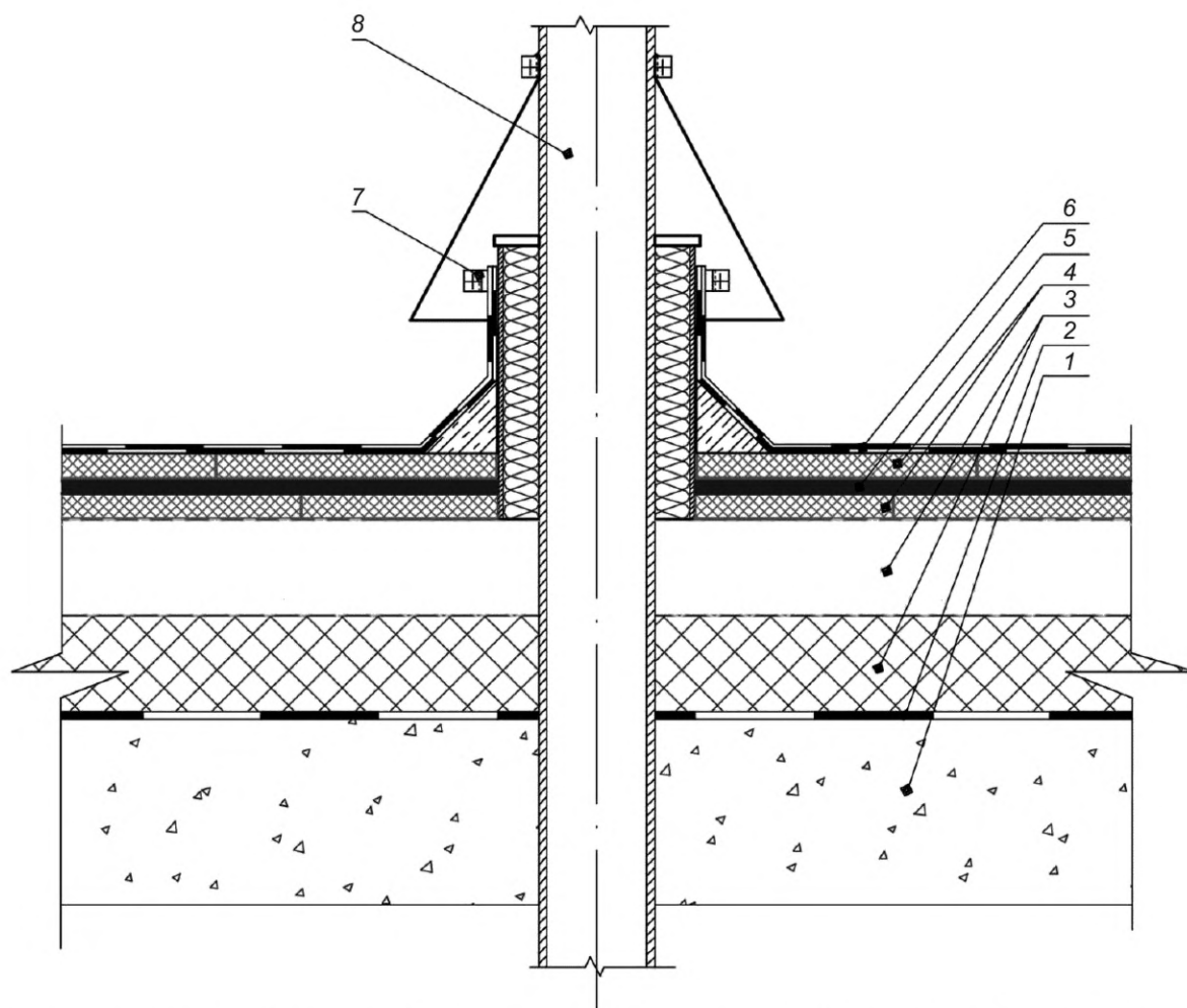
Рисунок В.2 — Схема монтажа слоя вблизи трубы
