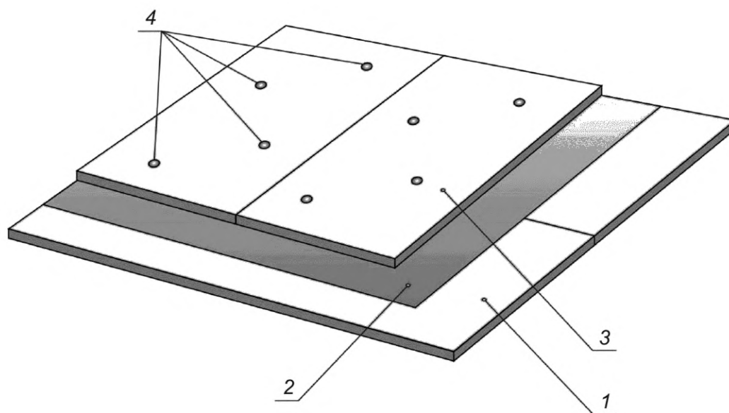
1 — нижний уровень листов сборной стяжки; 2 — электропроводящий рулонный материал, формирующий слой; 3 — верхний уровень листов сборной стяжки; 4 — механический крепеж
