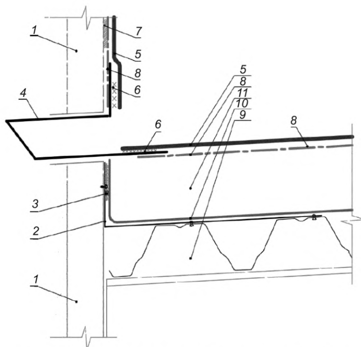
Рисунок Б.7 — Схема монтажа слоя вблизи слива через парапет
