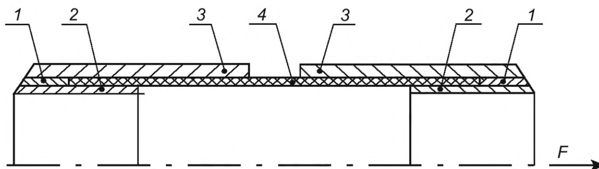
а) Образец с наконечником из листового проката
