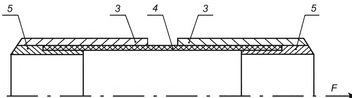
б) Образец из трубного наконечника
