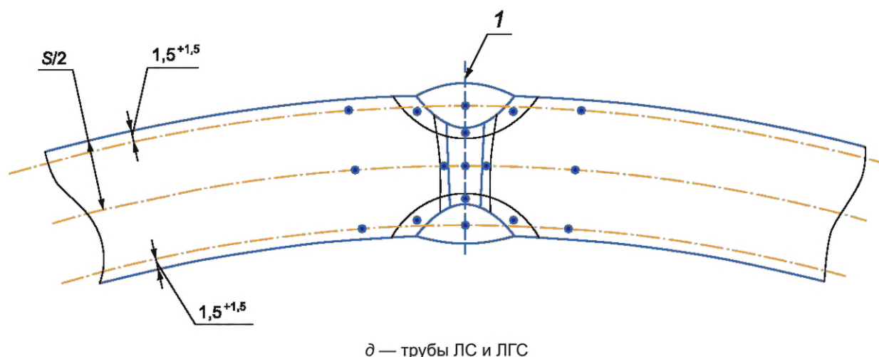
Рисунок 3, лист 2
