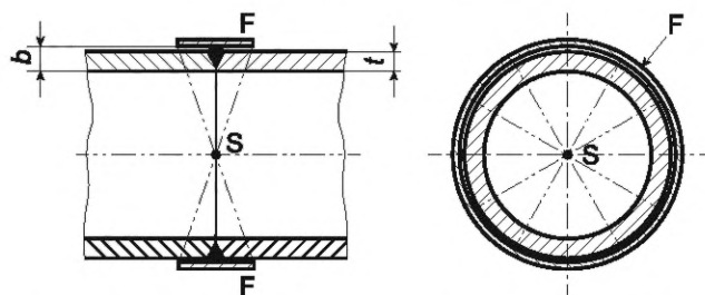
Рисунок 2 — Панорамная схема. Применяется для контроля объектов изогнутой формы при просвечивании через одну стенку
