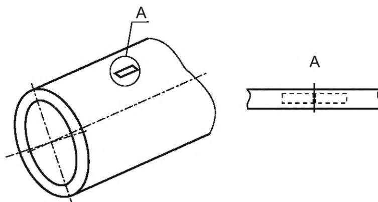
Рисунок 1 — Ориентация надреза на образцах для испытаний на ударный изгиб
