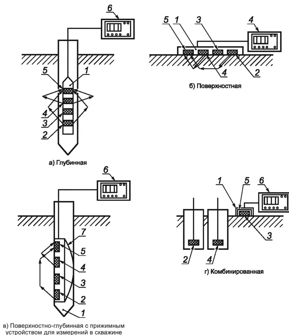
Рисунок 4 — Схемы измерений радиоизотопными влагоплотномерами
