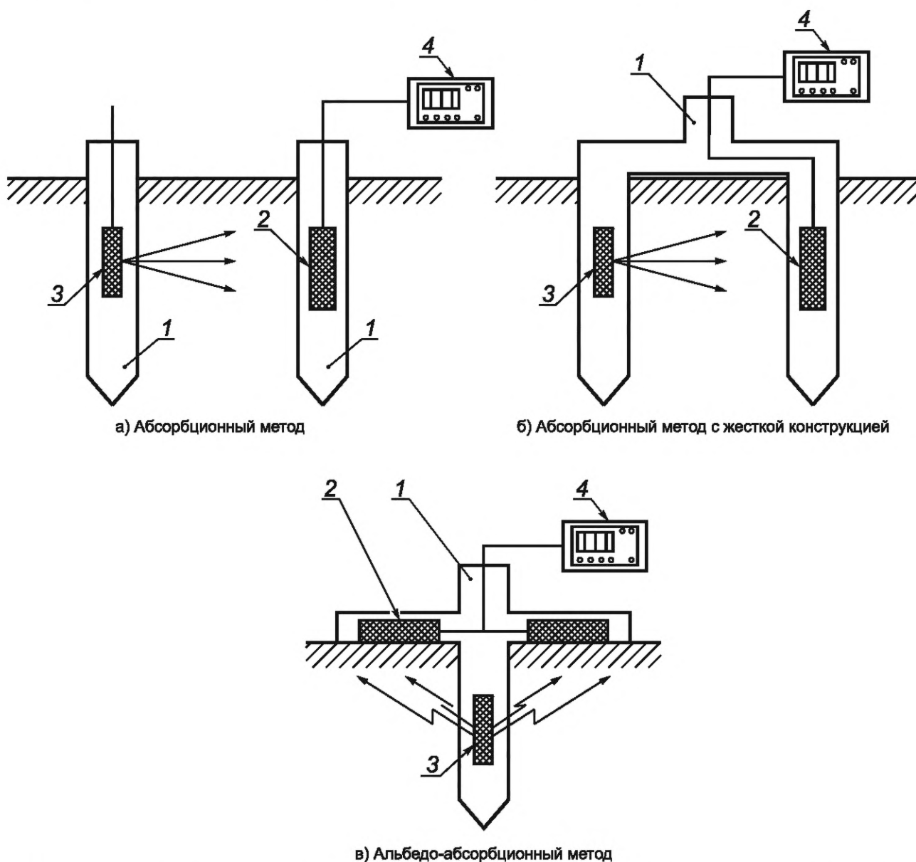
Рисунок 2 — Схемы измерений радиоизотопными плотномерами
