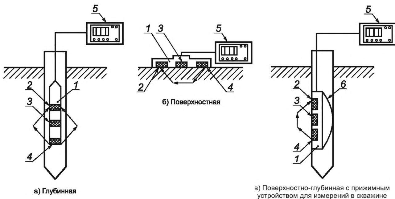
1 — измерительный преобразователь; 2 — детектор; 3 — защитный экран; 4 — радиоизотопный источник; 5 — измерительный прибор; 6 — прижимное пружинное устройство
