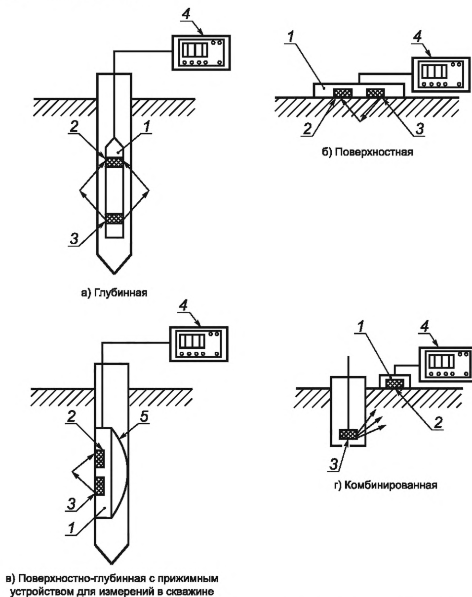
Рисунок 3 — Схемы измерений нейтронными влагомерами
