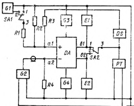
DA—КН; G1, G3, G4—источники постоянного напряжения; G2—генератор импульсов; DS—устройство выбора и хранения; PT—измеритель временных интервалов; E1, E2—эквиваленты нагрузки; R1—R4—резисторы; SA1, SA2—переключатели; a1—неинвертирующий вход КН; a2—инвертирующий вход КН; b1—неинвертирующий выход КН; b2—инвертирующий выход КН.
