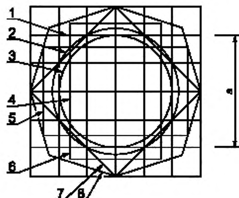
Рисунок 4.19 — Основная схема
