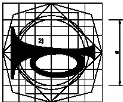
Рисунок 4.6 — Звуковой предупредительный сигнал
