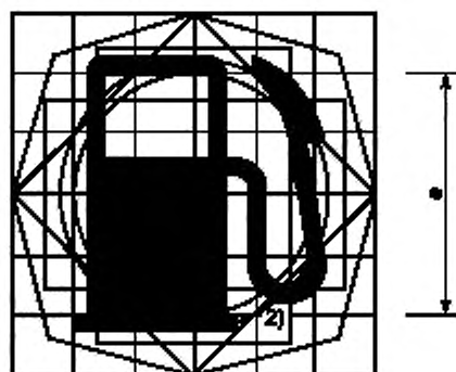
Рисунок 4.7 — Топливо
