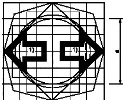
Рисунок 4.3 — Указатель поворота
