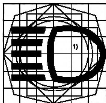
Рисунок 4.1 — Включение фар. Дальний свет
