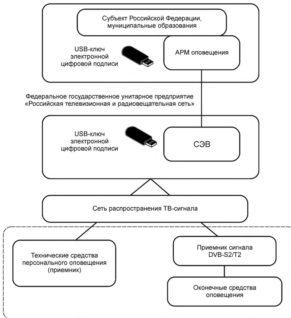
Рисунок В.2 — Схема взаимодействия АРМ оповещения и СЭВ для управления ОУ звукового, речевого и персонального оповещения
