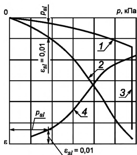
б) По схеме «двух кривых»
