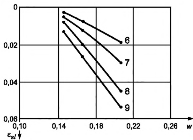
в) График зависимости относительной просадочности от влажности
