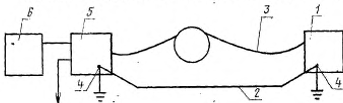
Расположение оборудования при измерении напряжения радиопомех
