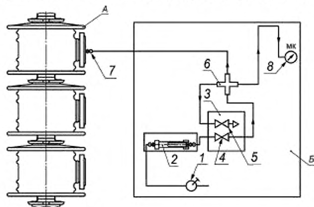
1 — насос; 2 — фильтр-влагодетелитель; 3 — блок кранов; 4 — запорный кран; 5 — кран сброса; 6 — коллектор; 7 — штуцер; 8 — тягонапоромер; А — колонка РПК; Б — прибор проверки герметичности
