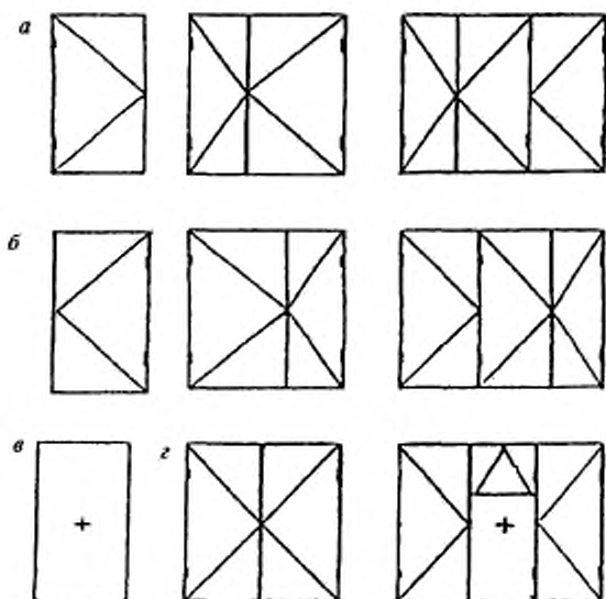
Рисунок А.2 — Определение изделий по направлению открывания створок
