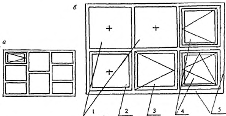
a — пример деревянной оконной рамы для остекления веранды; б — пример металлической рамы с различными видами заполнения конструкции: 1 — стеклопакетом; 2 — неоткрывающейся створкой (или остекленной коробкой); 3 — открывающейся (распашной) створкой; 4 — оконными блоками; 5 — рама
